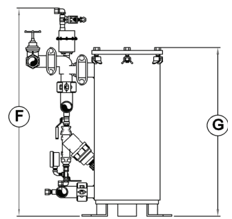
VISTA LATERAL
