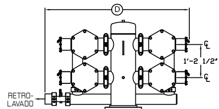
ELEVACION
